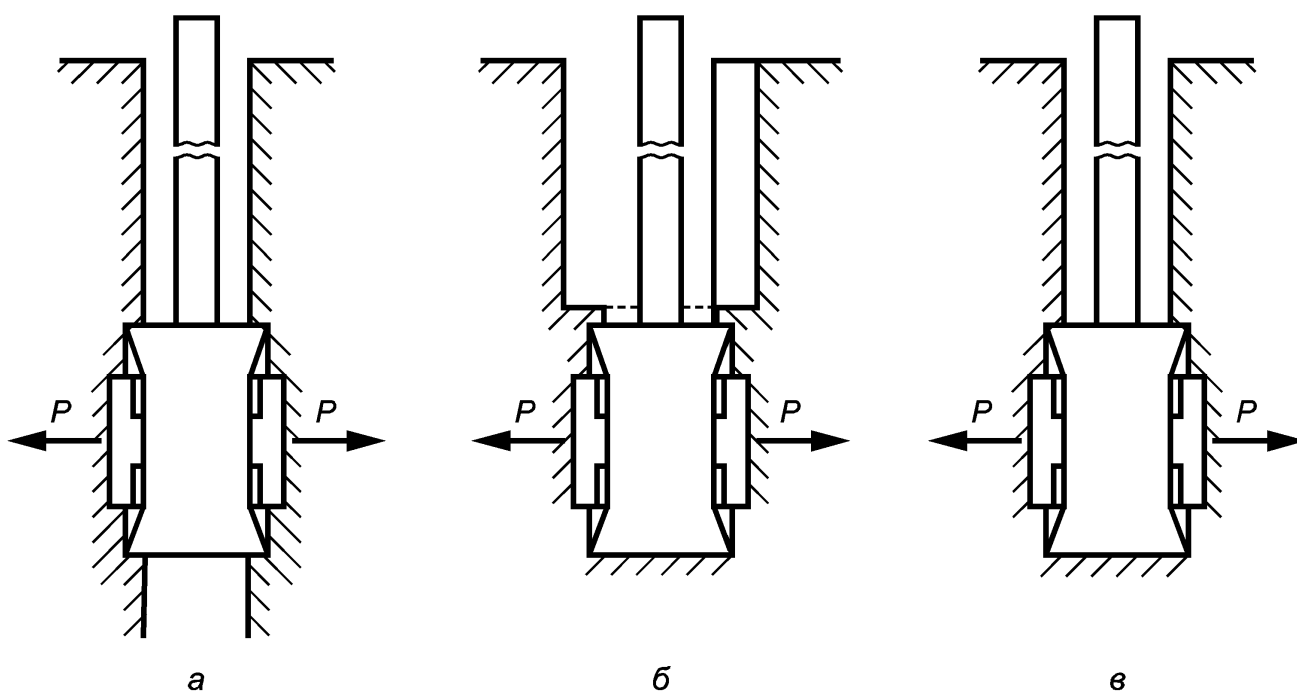
а - в стенках скважины; б - ниже забоя буровой скважины; в - в массиве
