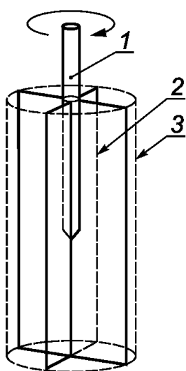
1 - штанга; 2 - лопасть; 3 - цилиндрическая поверхность среза
