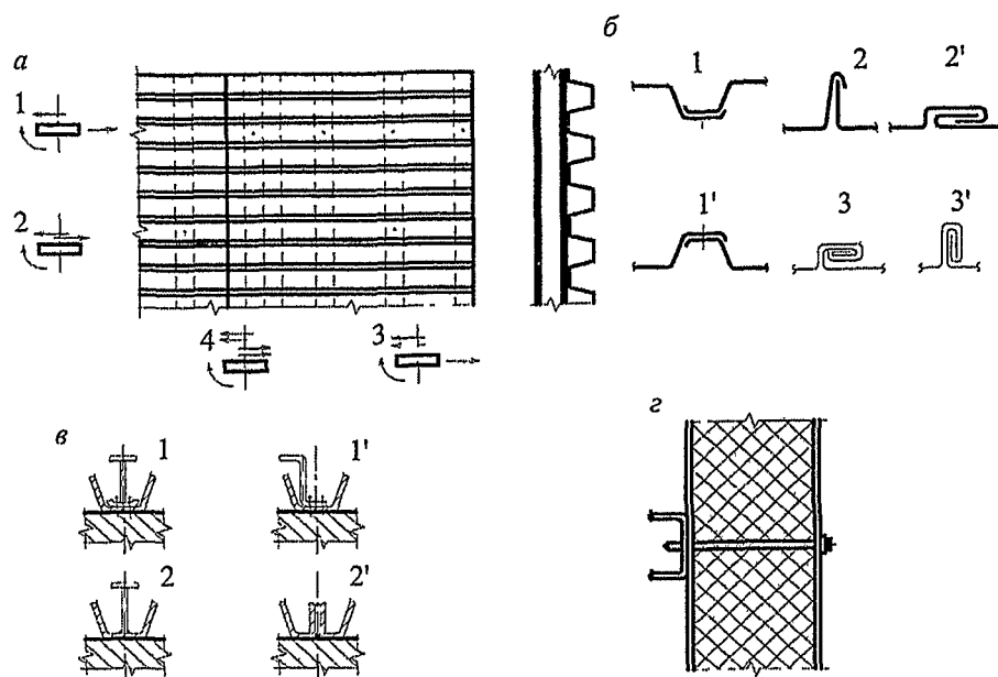
a – фрагмент конструкции покрытия со стальным профилированным настилом и схема действия сил на опорах (1– соединения в среднем участке; 2 и 3 – соединения соответственно по продольным и поперечным полкам; 4– соединения в месте пересечения продольных и поперечных полок); б – схема соединений по продольным полкам (1 и 1' – при расположении полок внахлест в нижнем и верхнем положениях соответственно для утепленных и холодных покрытий; 2 и 2' – простой стоячий и лежащий фальцы; 3 и 3' – двойной фальц, стоячий и лежащий); в – сдвигоустойчивые элементы (1 и 1' – на высокопрочных дюбелях; 2 – на контактной сварке; 2' – на дуговой сварке); z – фрагмент трехслойной стеновой панели на самосверлящем винте
