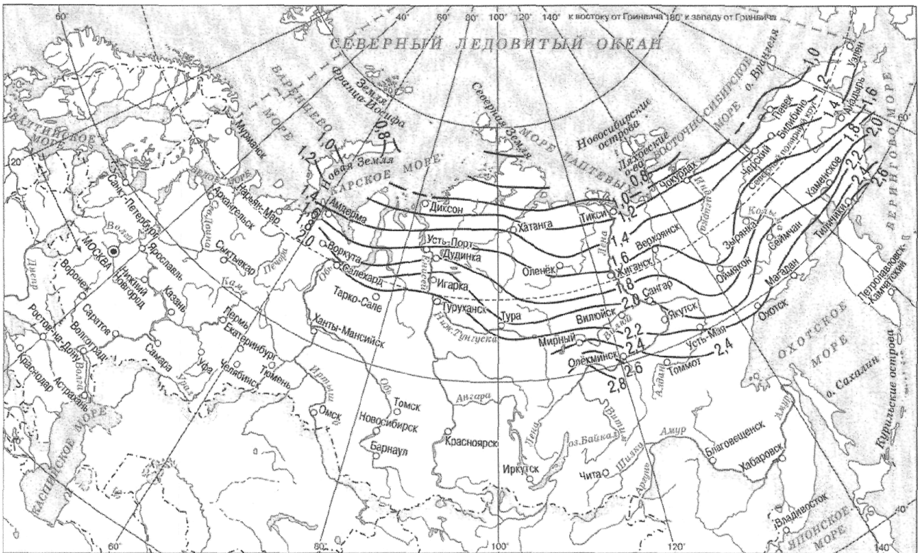
Рисунок Г.2 – Глубины оттаивания глинистых грунтов
