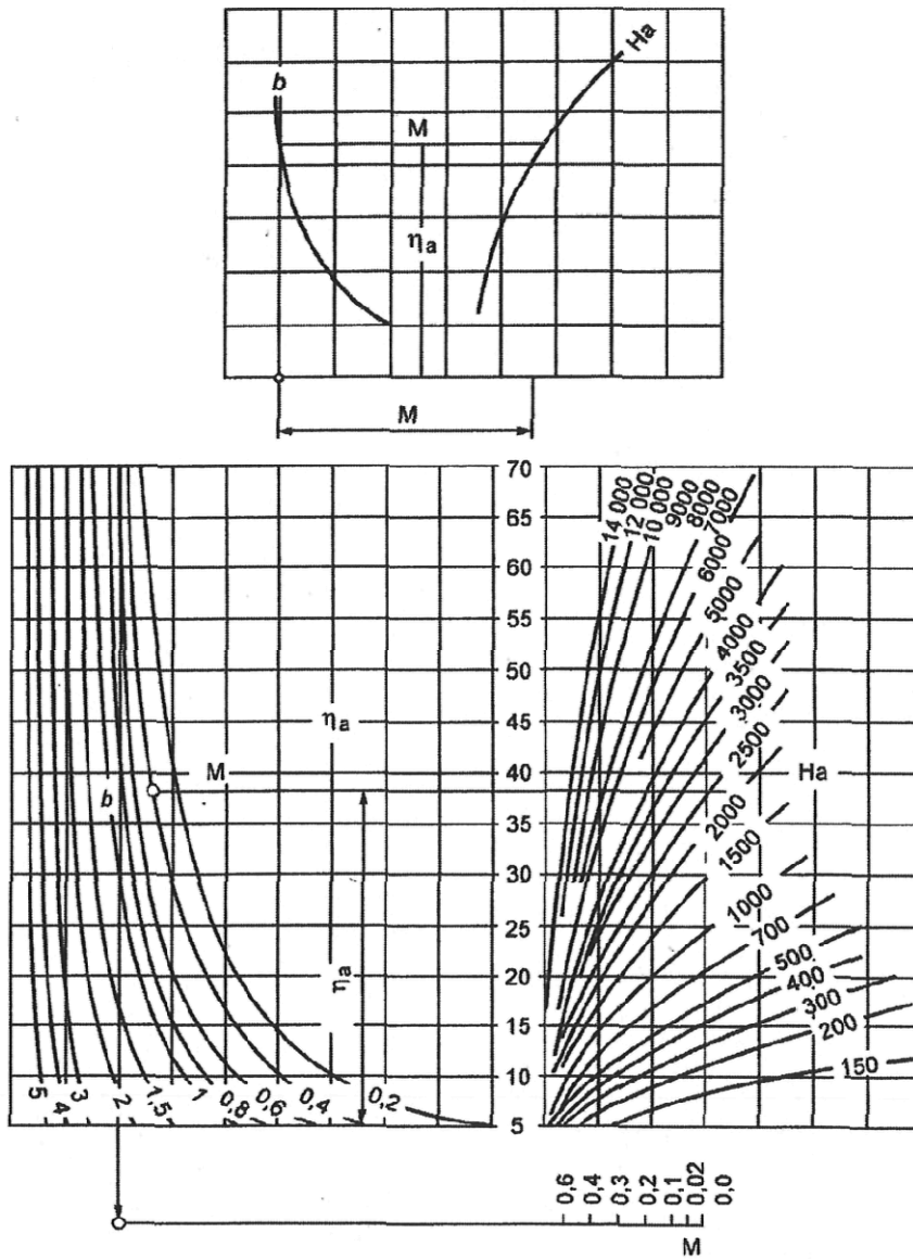
Рисунок P.1 – Номограмма для расчета радиуса охлаждения и оттаивания
