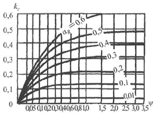
Рисунок К.1 – Графики для определения коэффициентов \xi_c и k_c
