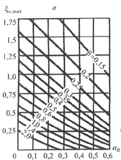
Рисунок К.3 – Графики для определения коэффициентов
