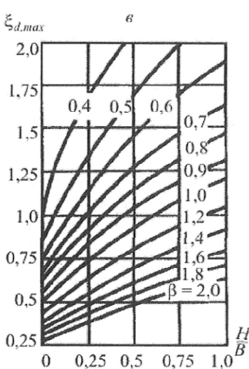
Рисунок К.3 – Графики для определения коэффициентов
