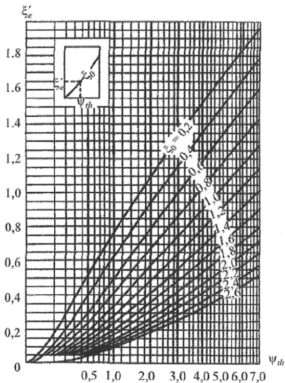
Рисунок К.6 – Графики для определения коэффициента \xi'e
