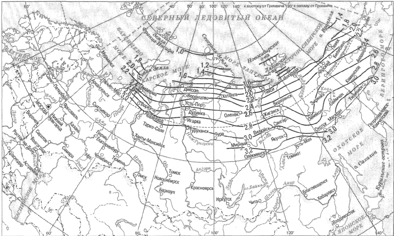
Рисунок Г.1 – Глубины оттаивания песчаных грунтов
