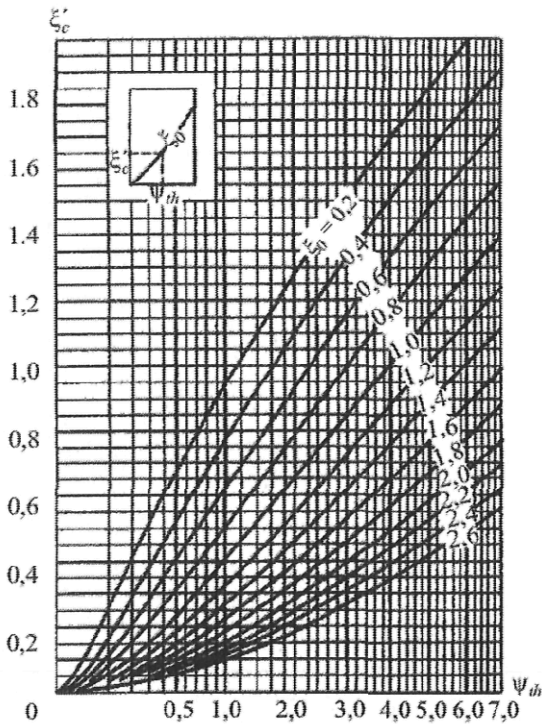
Рисунок К.5 – Графики для определения коэффициента \xi'_c
