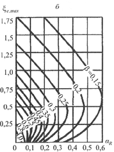
а – \xi_{c,max} ; б – \xi_{e,max} ; в – \xi_{d,max}
