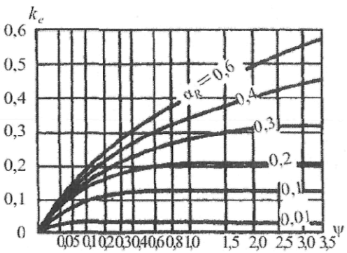
Рисунок К.2 – Графики для определения коэффициентов \xi_c и k_e
