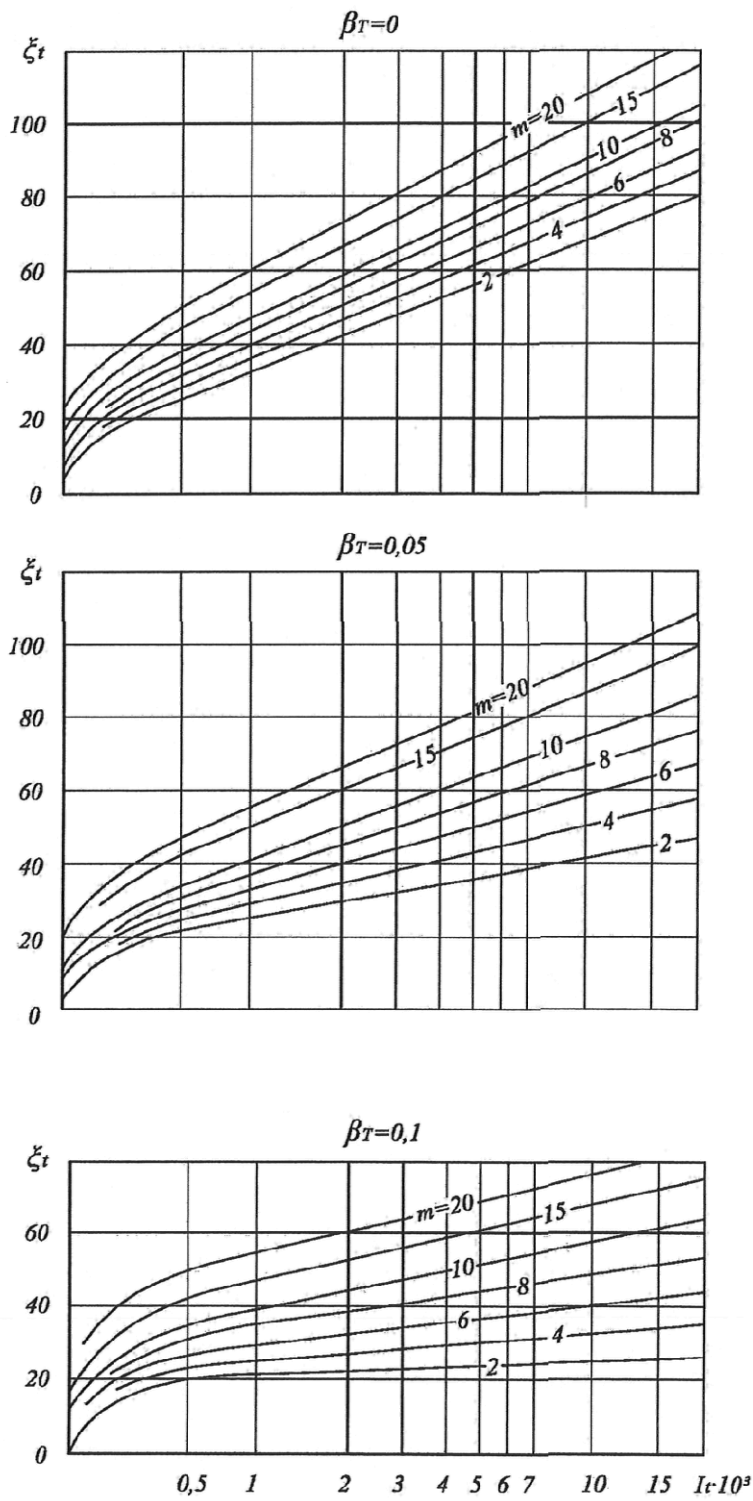
Рисунок Н.2 – Номограмма для определения многолетнего оттаивания многолетнемерзлых грунтов вокруг теплового и горячего трубопроводов
