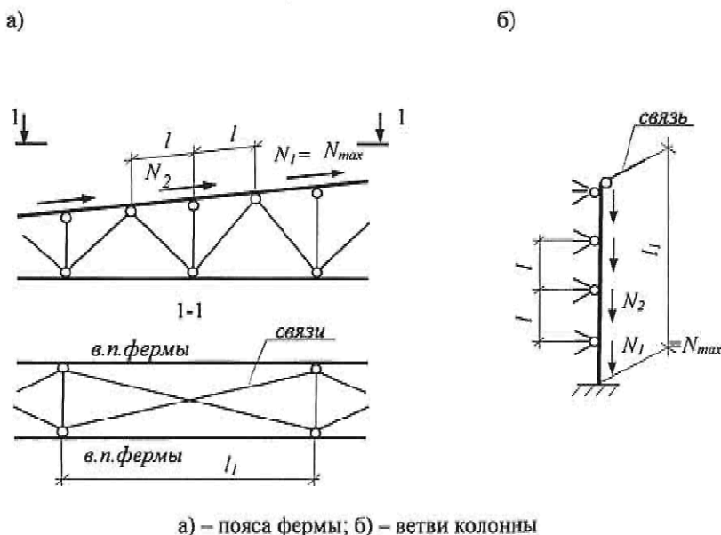
Рисунок 14 – Схемы для определения расчетной длины элементов
