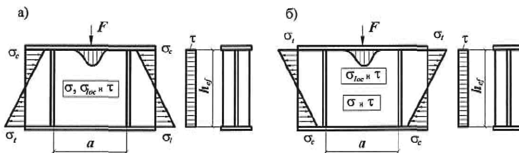
а) – при приложении сосредоточенной нагрузки к сжатому поясу; б) – то же, к растянутому поясу Рисунок 8 – Схема участка балки, укрепленной поперечными ребрами жесткости
