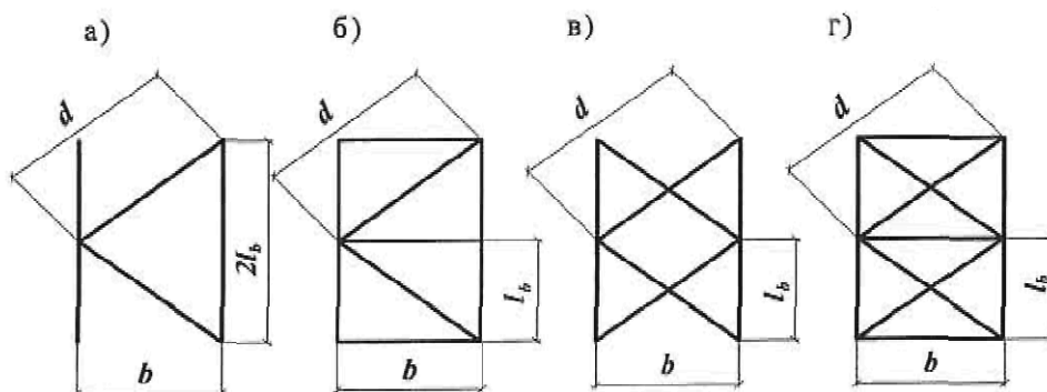
а) – треугольная; б) – треугольная с распорками; в) – крестовая; г) – крестовая с распорками
