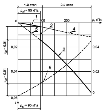
1 и 2 — зависимости относительного сжатия грунта от давления при природной влажности и водонасыщенном состоянии соответственно; 3 — относительное сжатие в результате замачивания — относительная просадочность грунта \epsilon_{pj} при p = 100 кПа; 4 и 5 — экстраполируемые кривые относительного сжатия грунта соответственно при природной влажности и водонасыщенном состоянии; 6 — кривая зависимости относительной просадочности \epsilon_{pj} от давления на грунт p , p_{0j} — начальное просадочное давление, принимаемое при \epsilon_{pj} = 0,01
