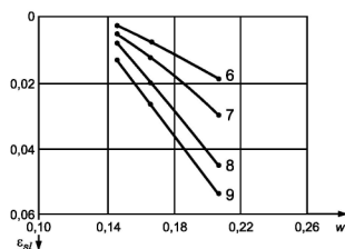
в) График зависимости относительной просадочности от влажности
