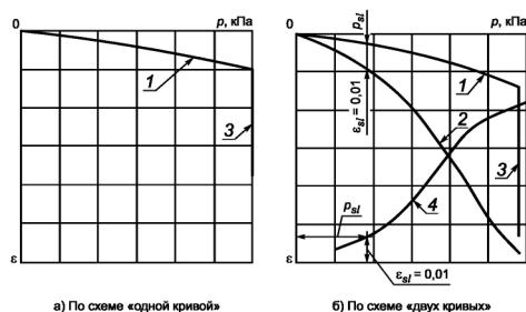
1, 2 — относительное сжатие \varepsilon грунта с природной влажностью и в водонасыщенном состоянии \varepsilon_w в зависимости от давления; 3 — дополнительное относительное сжатие грунта в результате замачивания (относительная просадочность \varepsilon_d ) при заданном давлении p_d ; 4 — зависимость относительной просадочности \varepsilon_d от давления; p_d — начальное просадочное давление
