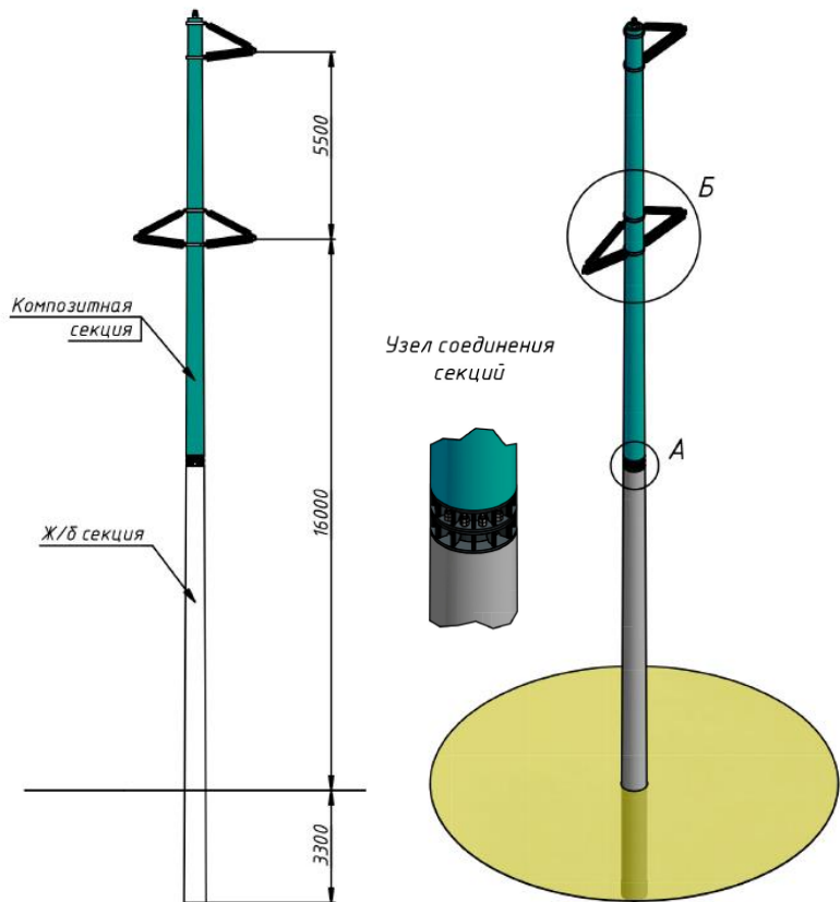
Вариант опоры 220 кВ с изолирующими траверсами Техническое решение
