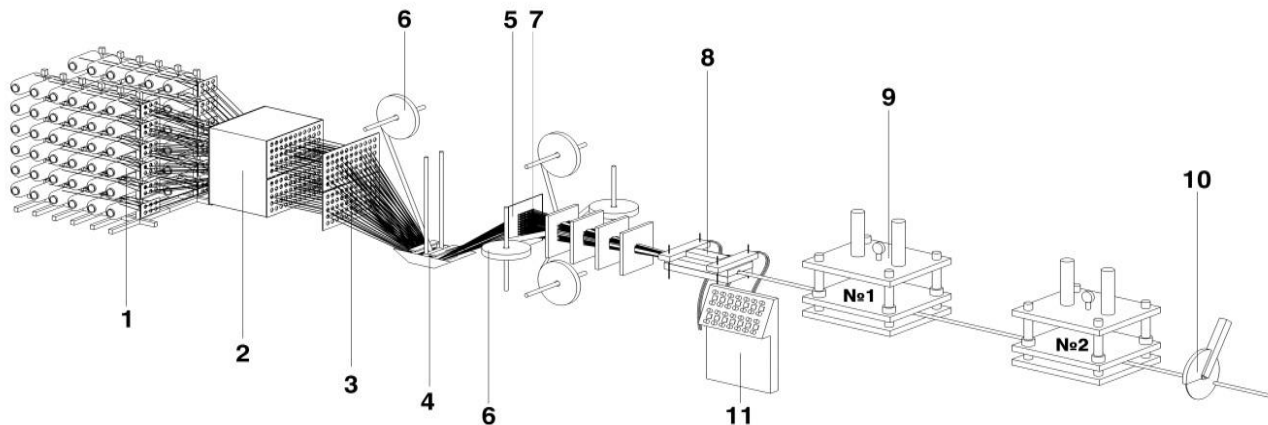
Схема пултрузионной установки
